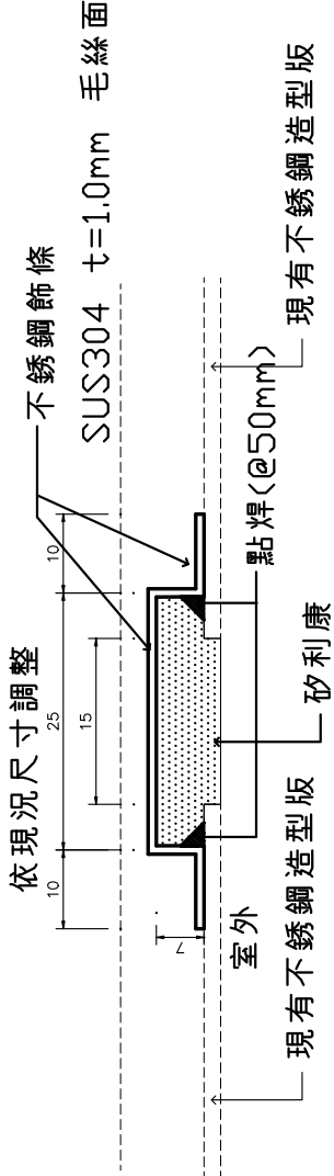
line ① ~ ⑰ 橫剖詳細圖 S=1/1
