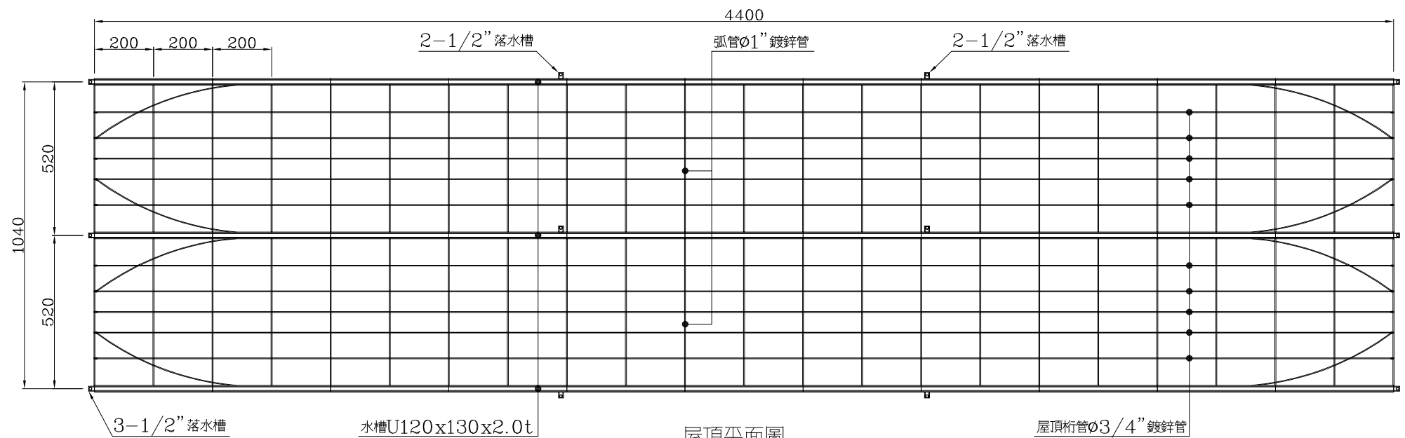
屋頂平面圖
