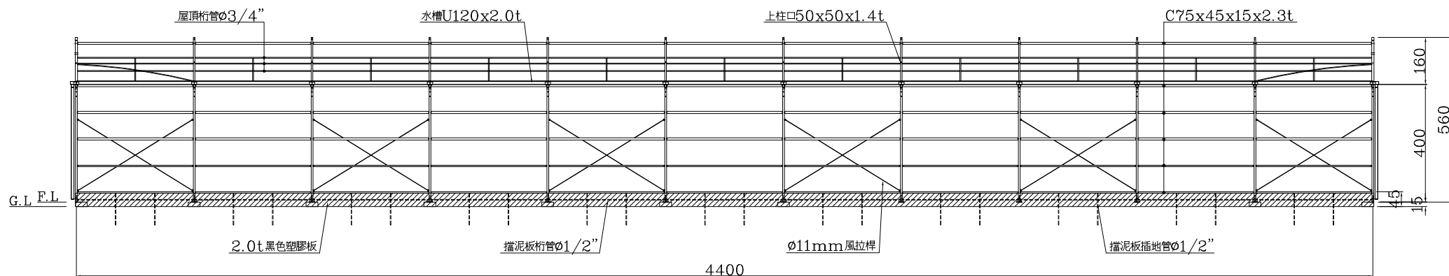
右側立面圖
