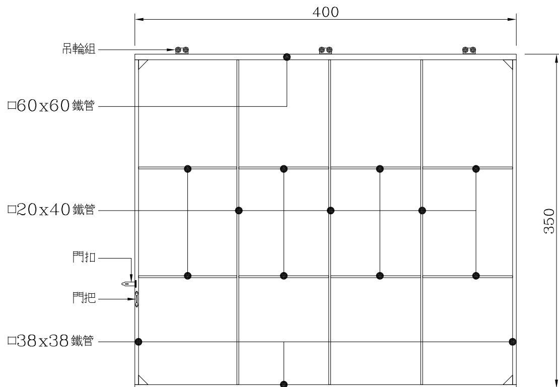
D2 單開鐵管吊門 400x350cmx1腔
