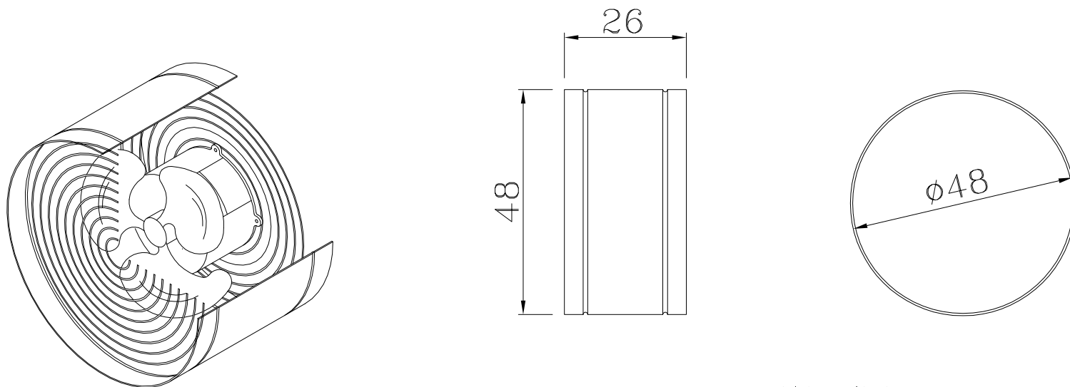
外框詳圖
