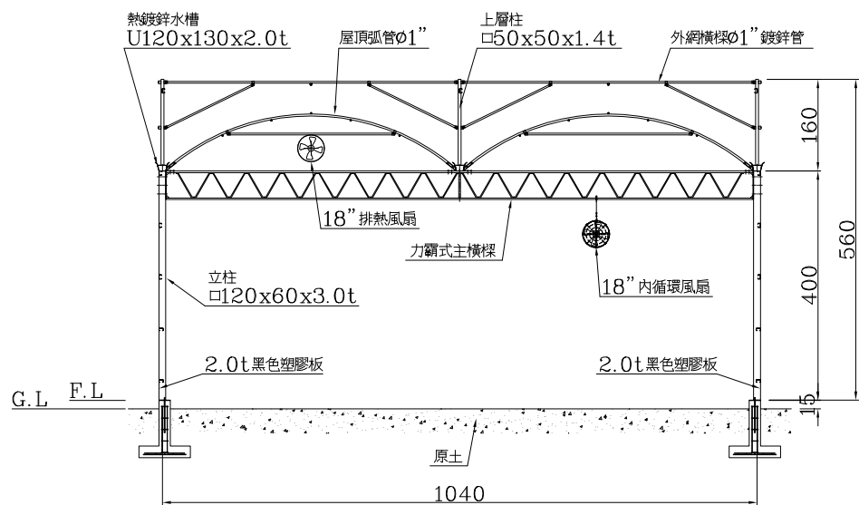
橫向剖面圖
