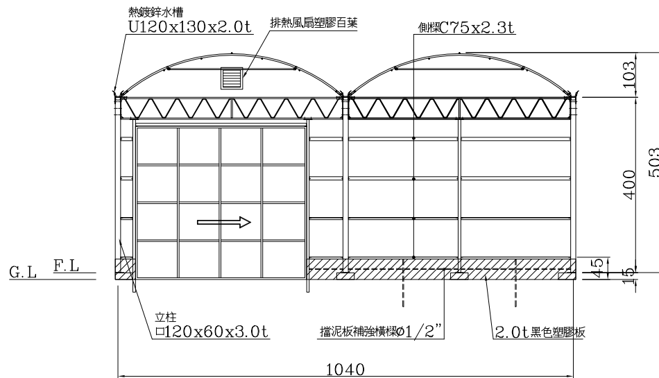
正向立面圖
