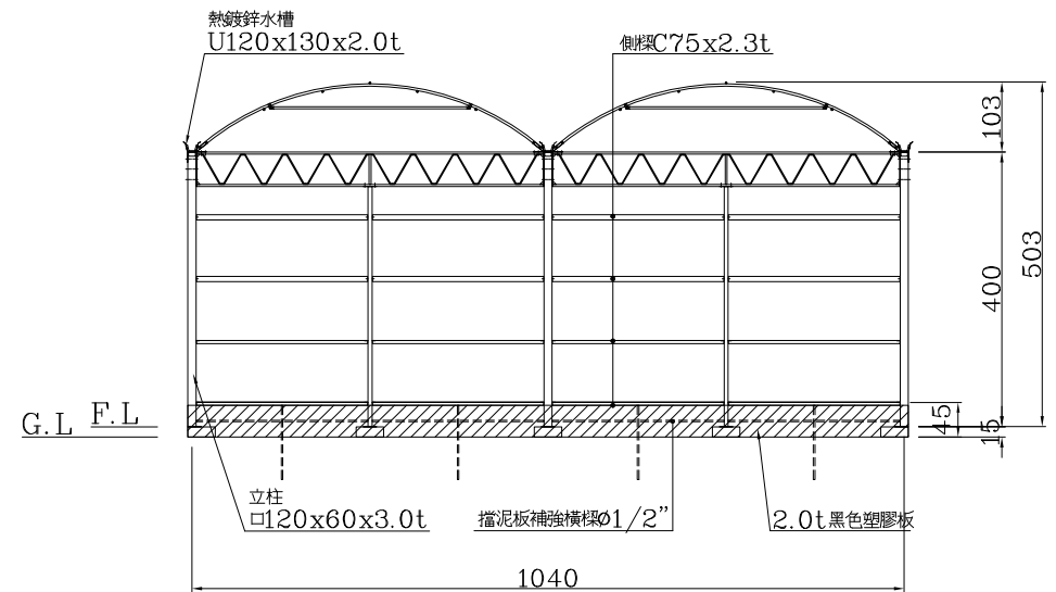
背向立面圖
