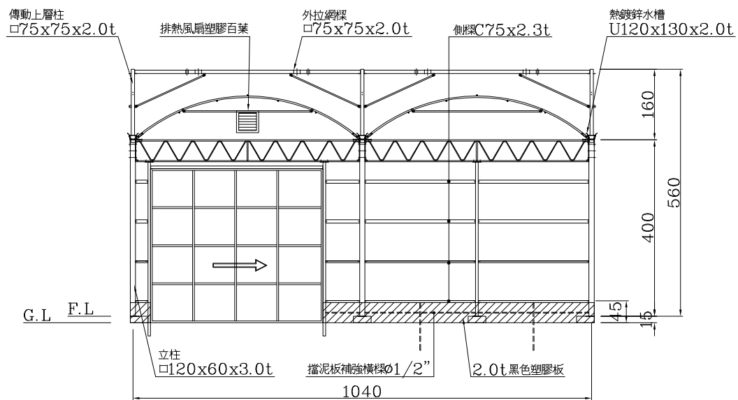
正向立面圖
