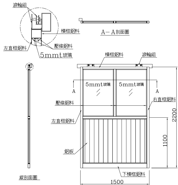
D1 單開玻璃鋁吊門 150x220cmx1腔
