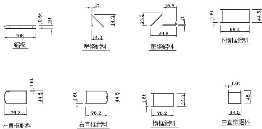
D1 單開玻璃鋁吊門 150x220cmx1腔
