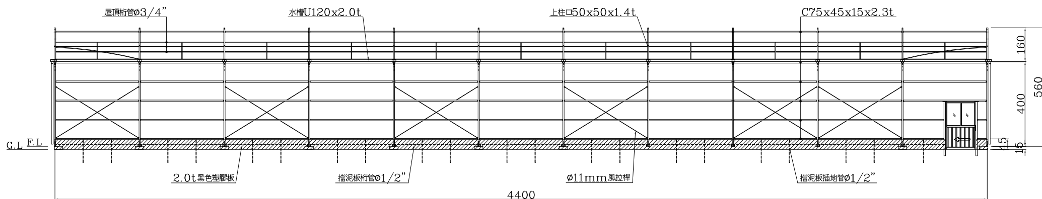
左側立面圖
