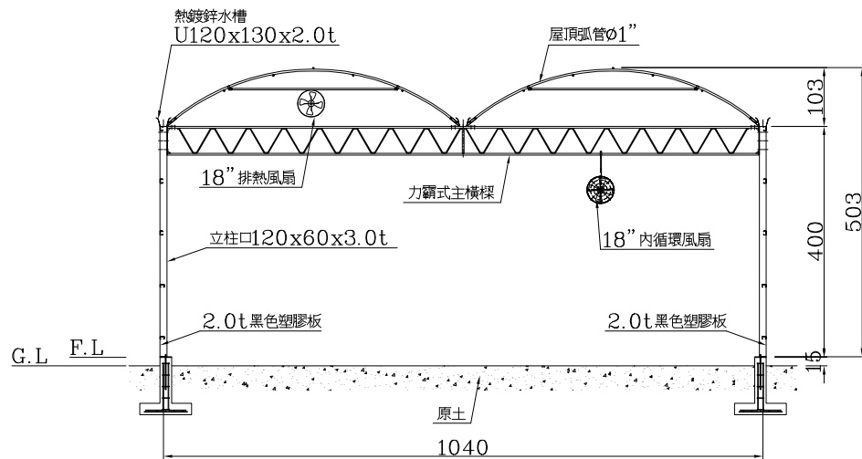
橫向剖面圖
