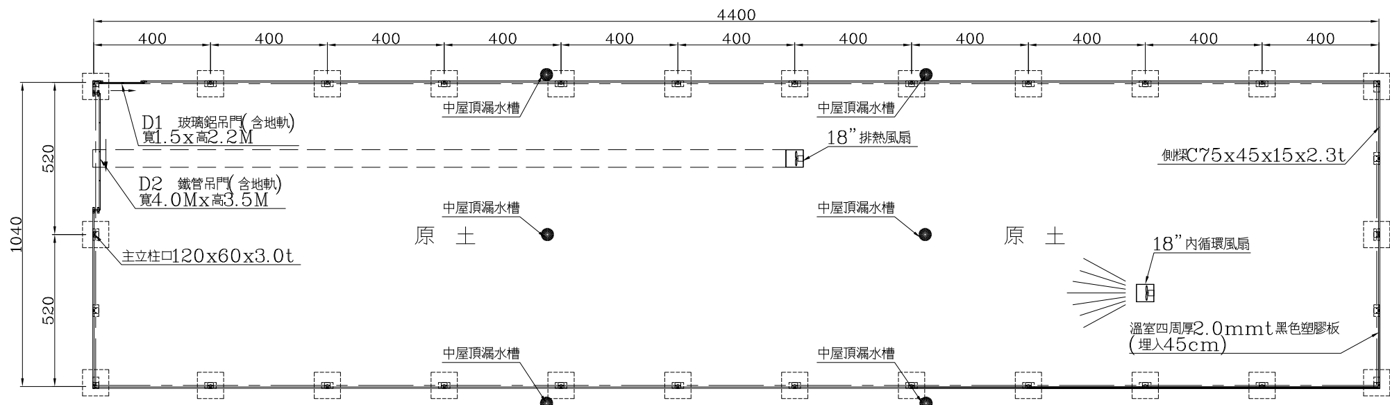
壹層平面圖
