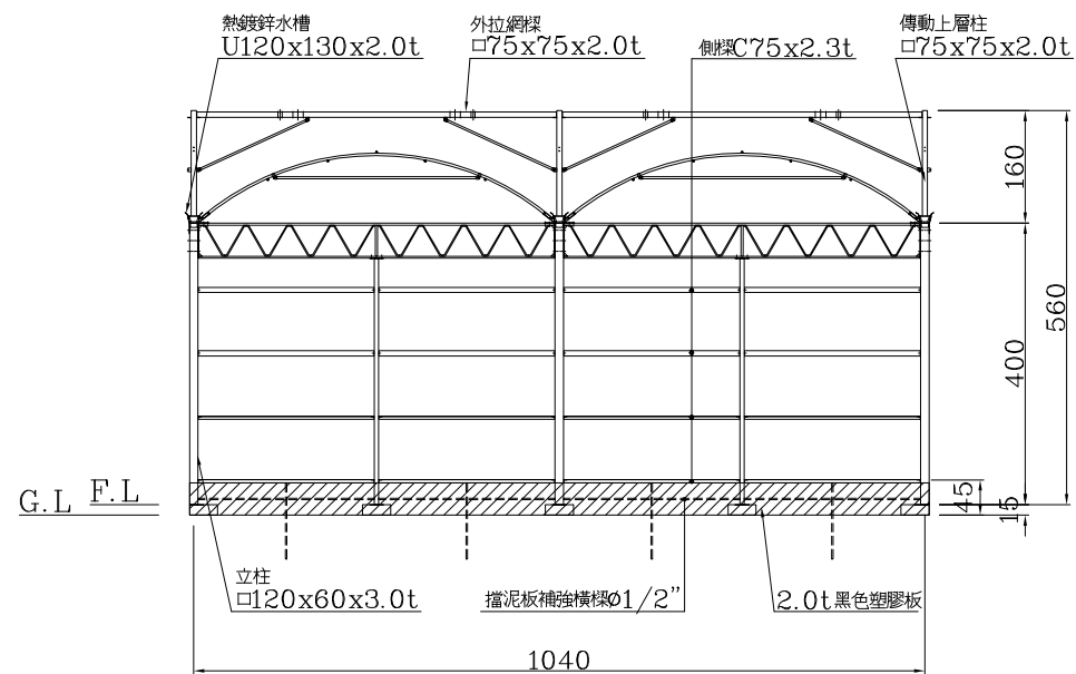
背向立面圖
