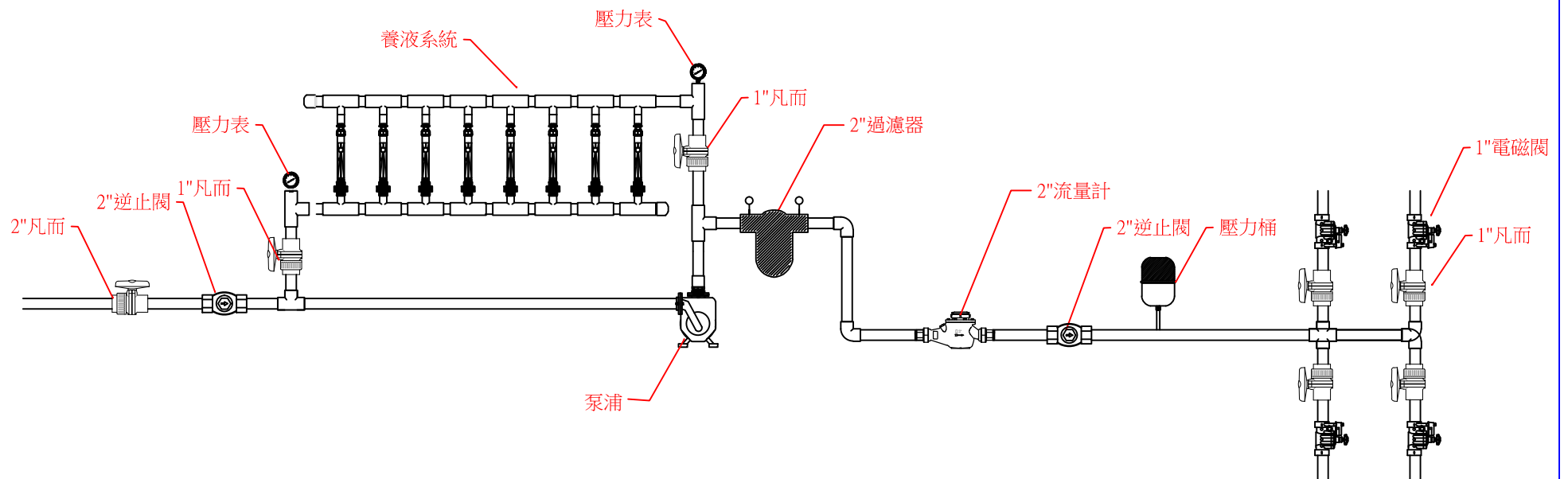
附件二 養液系統及分區灌溉系統流程圖
