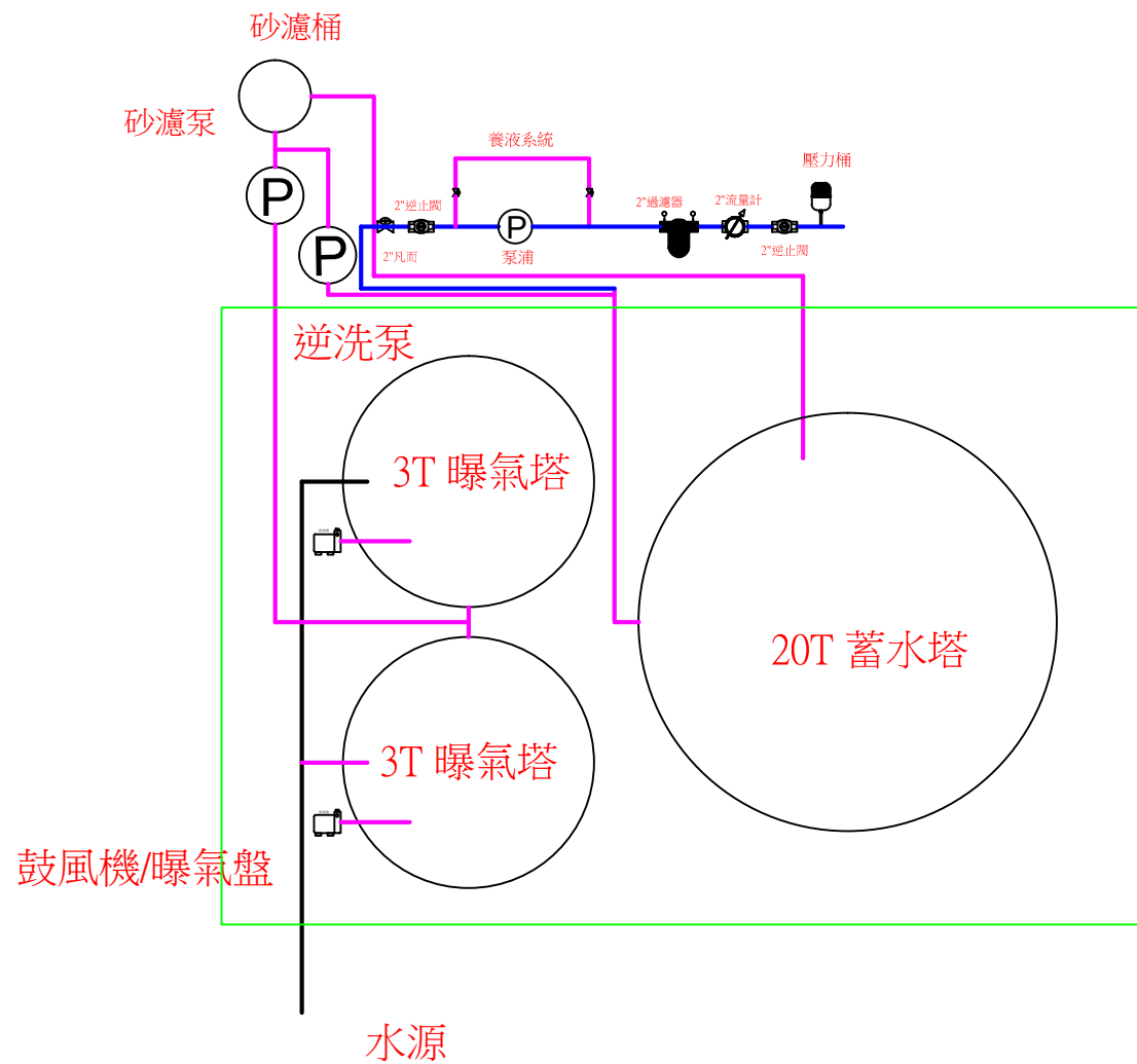
附件三 系統配置圖
