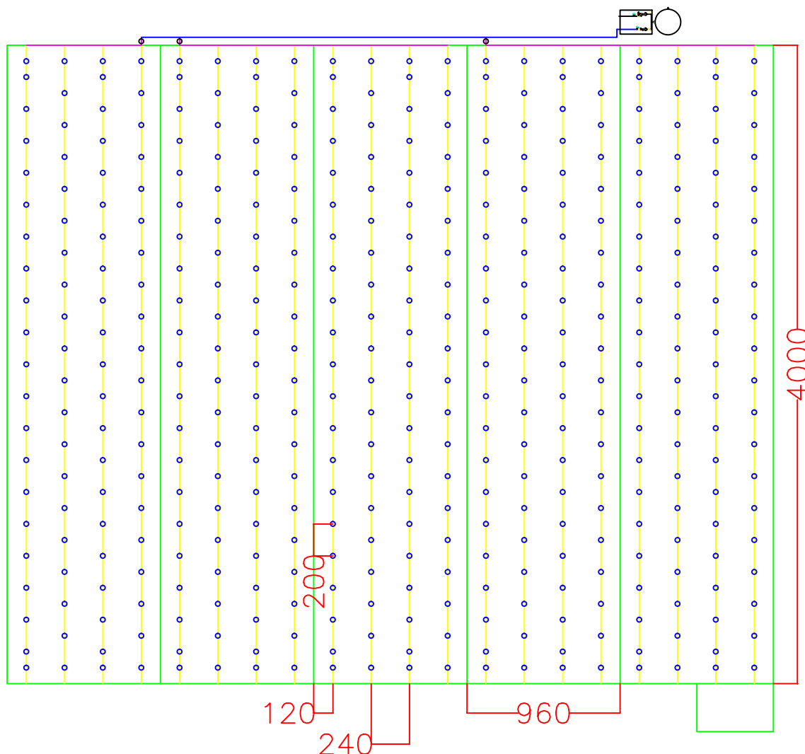
附件一 溫室噴霧系統配置圖
