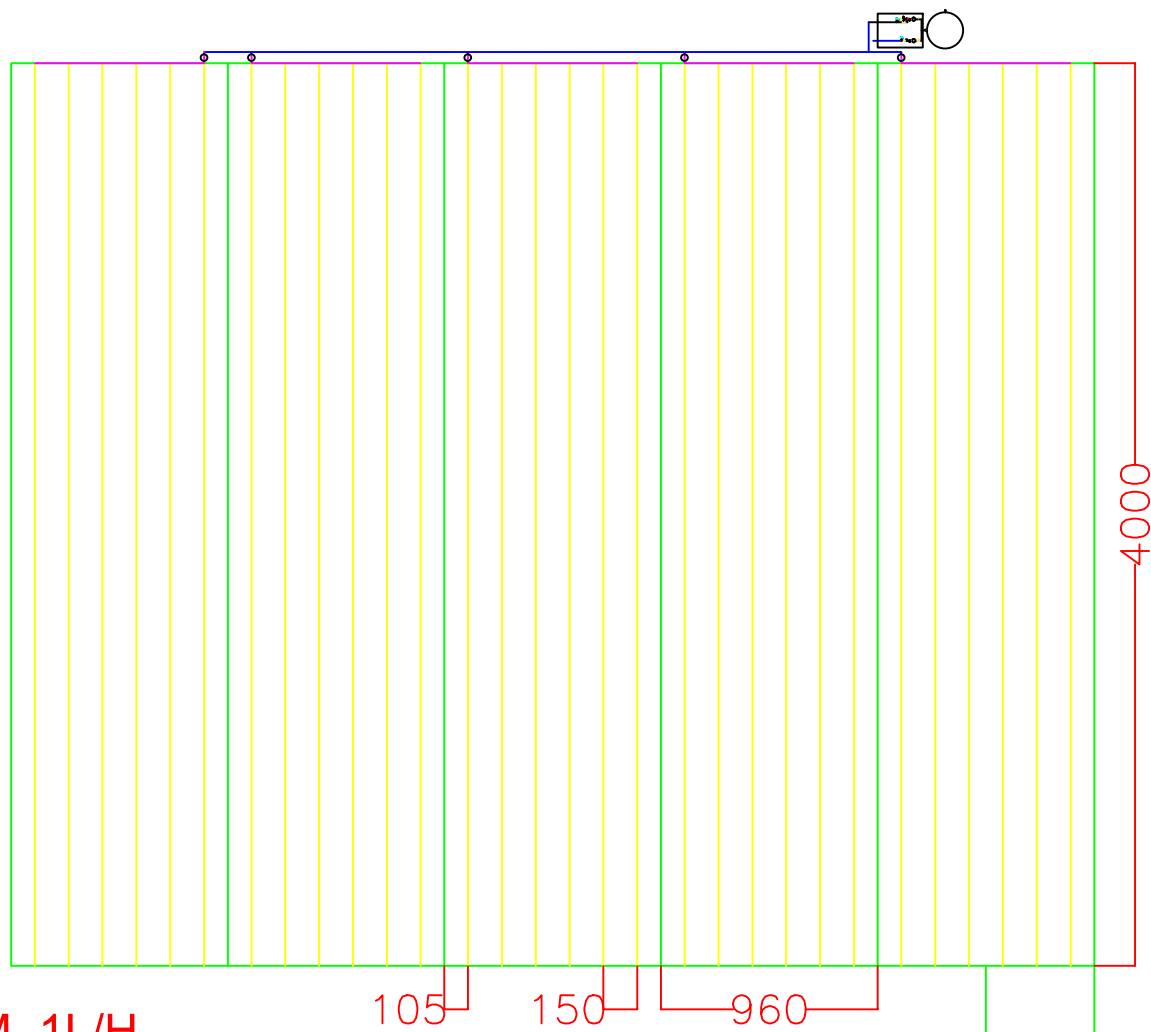
附件二 溫室滴灌系統配置圖
