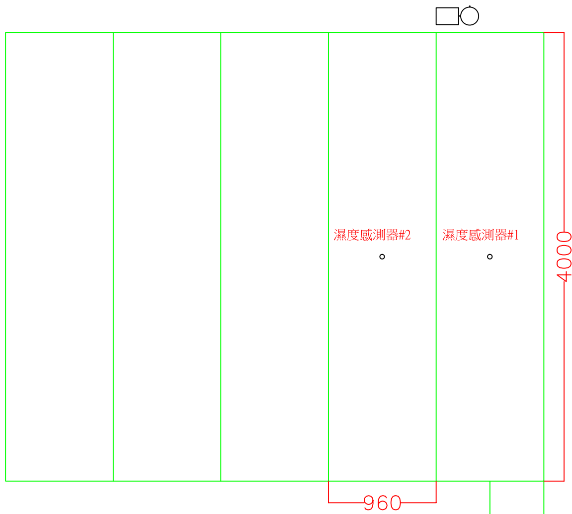
附件四 土壤濕度感測器配置圖
